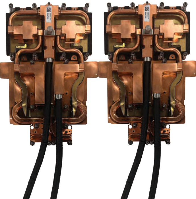
VS 传统 NVIDIA Blackwell 散热方案
